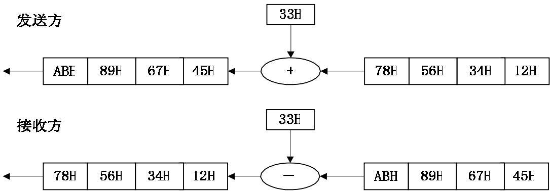
图9 传输次序图
