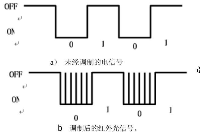
图5 信号与调制
